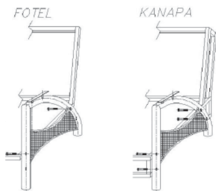
Poręcz mocowana bezpośrednio śrubami
